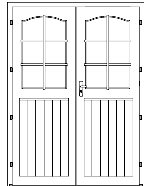
Doppeltür 70 mm ISO 1425 x 1955 mm 1 st.
