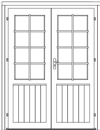
Doppeltür 40 mm 1425 x 1900 mm 1 stk.
