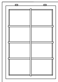
Fenster 40 mm 865 x 1210 mm 2 stk.
